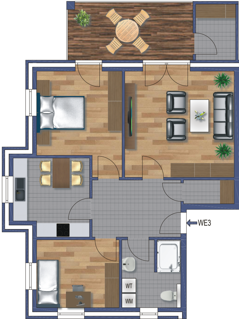
Dachgeschoss
